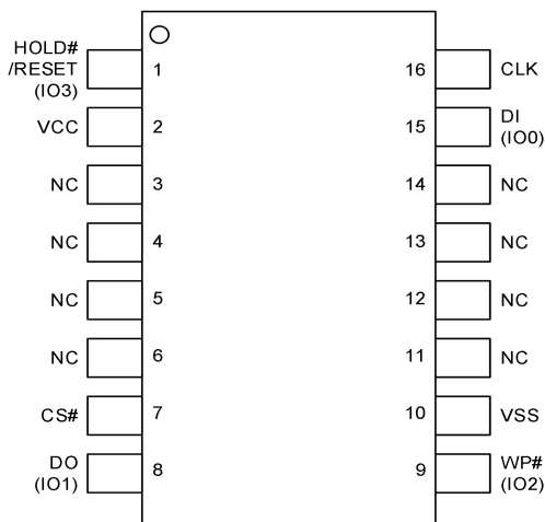
SOP16 300mil
